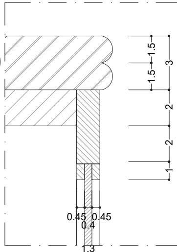
D1 Detail ML 5.03 1:2
