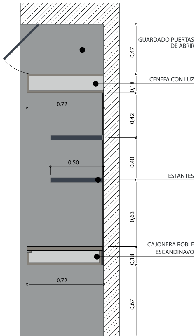
CORTE 2 ESC.1:20
