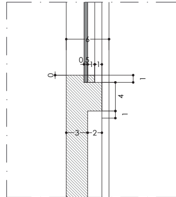
D.2 Detail 02 R-CA03 1:5
