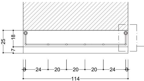
P Plan ML 5.03 1:20
