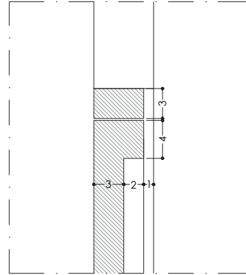
D.3 Detail 03 R-CA03 1:5
