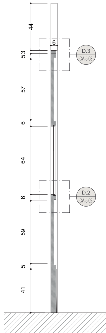
S.1 Section R-CA03 1:20
