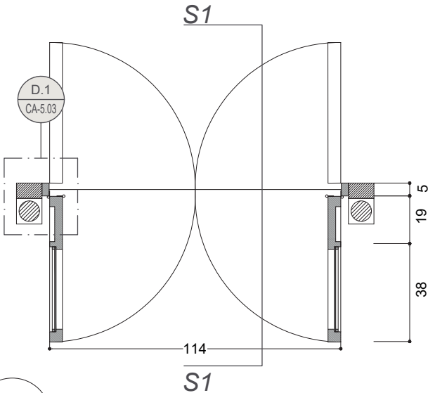
P.1 Plan R-CA03 1:20
