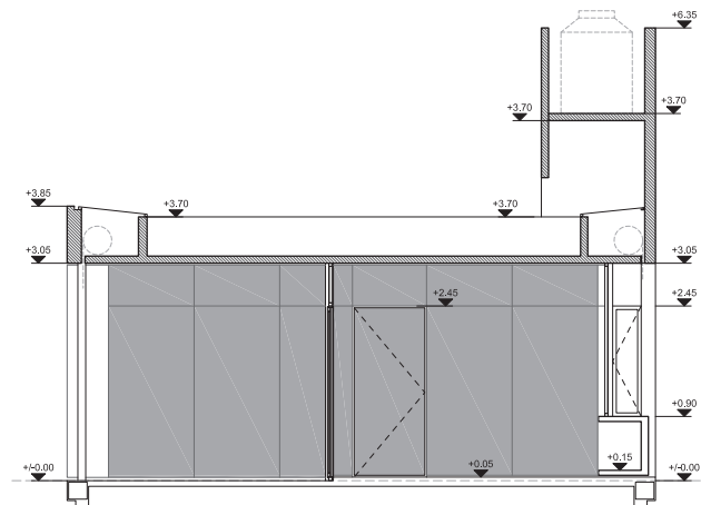
Corte B-B
