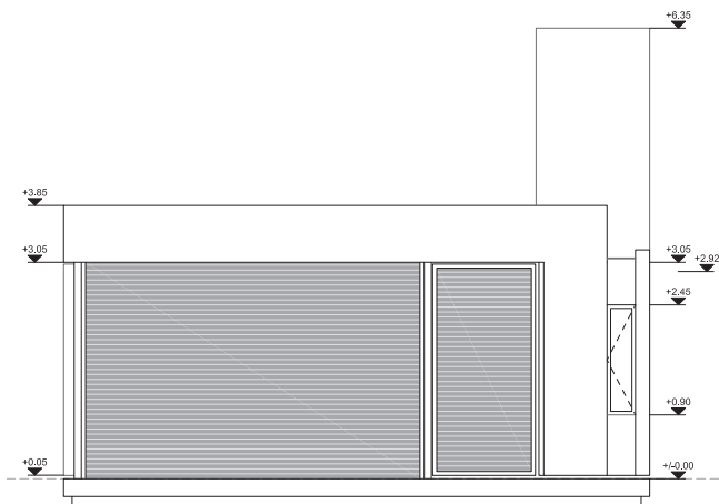
Vista Sur
