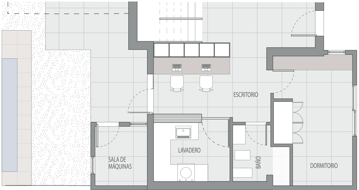
Planta Lavadero | Escritorio ⌀
