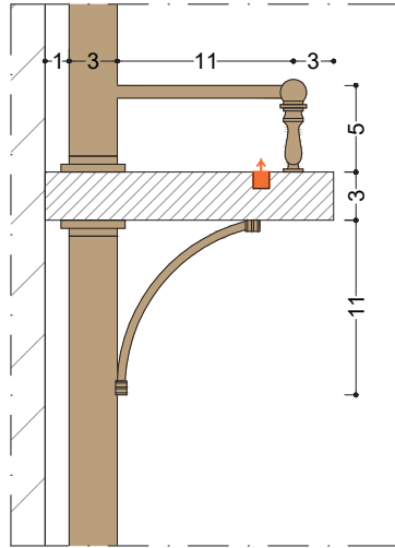
D2 Detail ML 5.03 1:5
