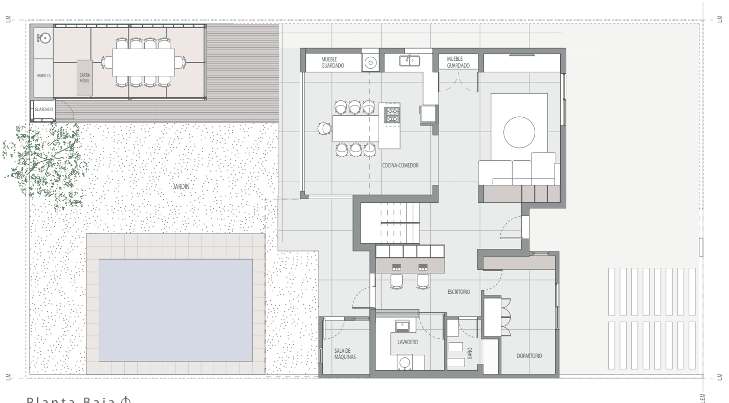
Planta Baja ⌚
