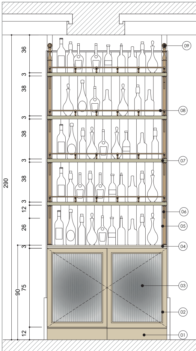
E Elevation ML 5.03
