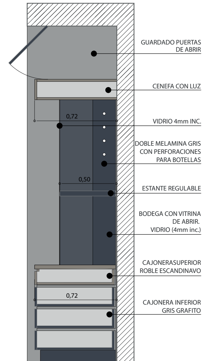
CORTE 1 ESC.1:20
