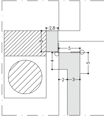
D.1 Detail 01 R-CA03 1:5
