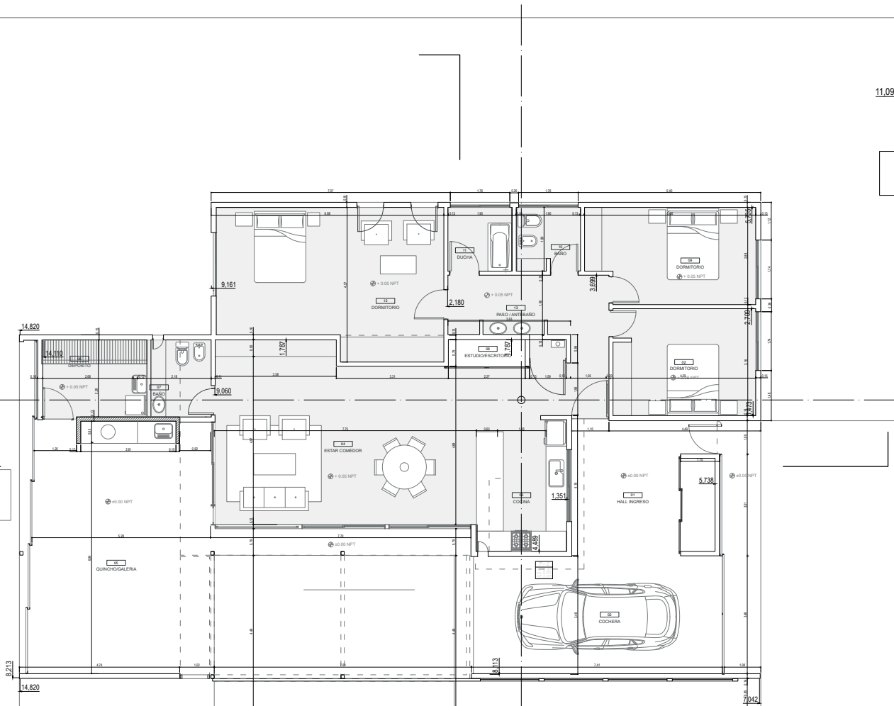
Planta General ⊕
